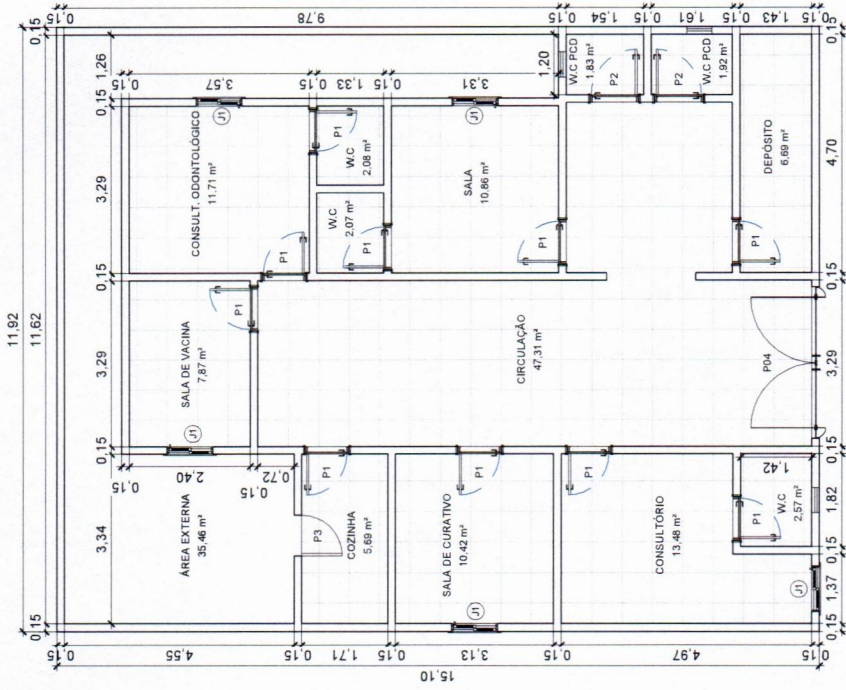
1 PLANTA BAIXA 1 : 100
