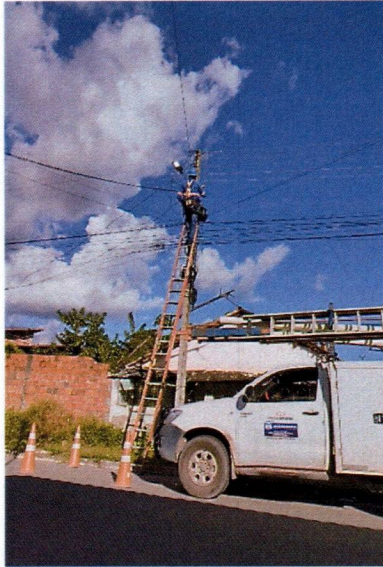
Figura 05: equipe em campo realizando substituições necessárias de Lâmpadas, cabo elétrico, conector, reator, arruela, braços com caminhonete adaptada.
