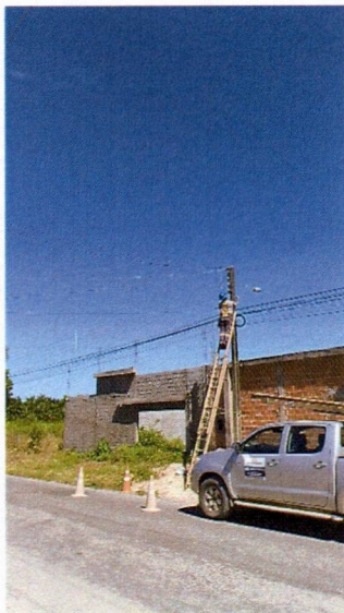
Figura 07: equipe em campo realizando substituições necessárias de Lâmpadas, cabo elétrico, conector, reator, arruela, braços com caminhonete adaptada.
