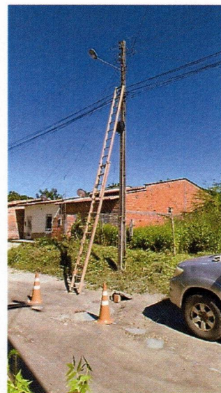
Figura 06: equipe em campo realizando substituições necessárias de Lâmpadas, cabo elétrico, conector, reator, arruela, braços com caminhonete adaptada.
