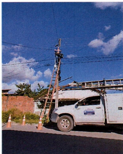
Figura 01: equipe em campo realizando substituições necessárias de Lâmpadas, cabo elétrico, conector, reator, arruela, braços com caminhonete adaptada.
