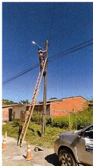
Figura 06: equipe em campo realizando substituições necessárias de Lâmpadas, cabo elétrico, conector, reator, arruela, braços com caminhonete adaptada.
