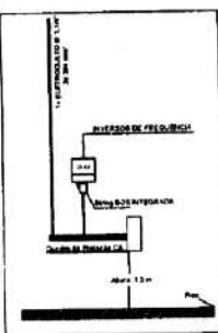
DETALHE 1 - Instalação dos Inversores
